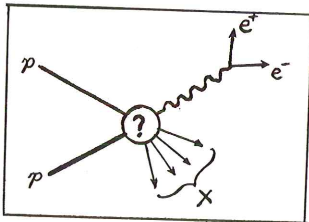
圖二： p + p \rightarrow e^+ + e^- + X 的反應。曲線表示虛光子。
