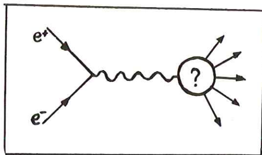
圖三：正負電子湮滅。曲線表示虛光子。
