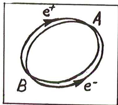
圖四：正負電子在存儲環示意圖。A,B兩點為碰撞區域。
