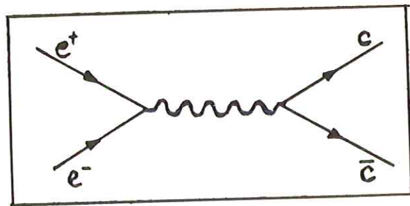
圖五：產生 c\bar{c} 的費曼圖。
